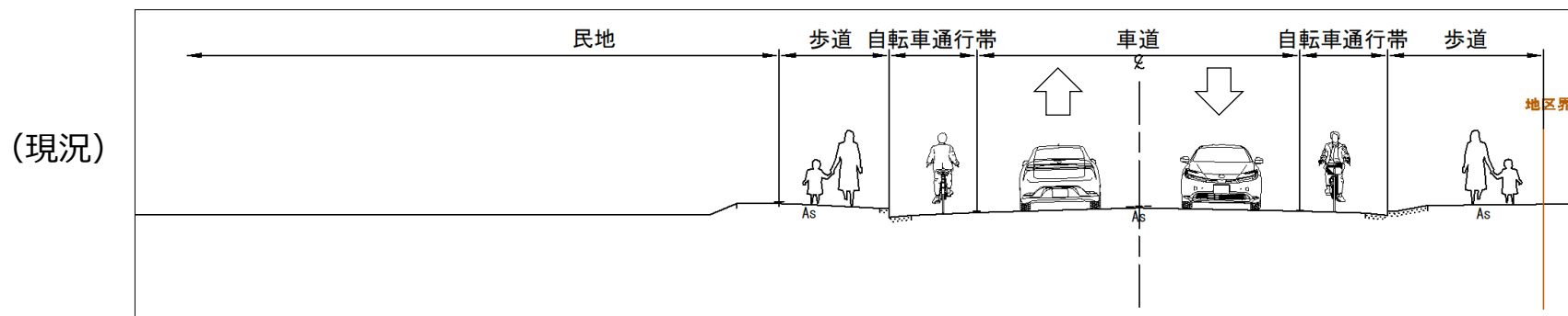
施工図②：断面図
