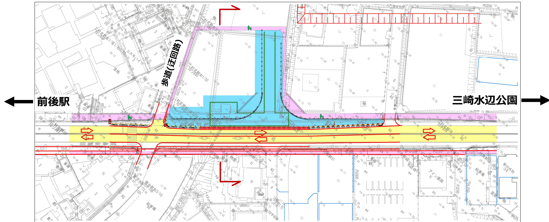
施工図③：平面図
